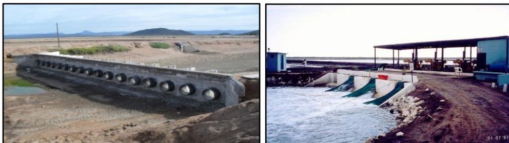
Fotos 73 e 74 – Filtração primária no canal de abastecimento de fazenda de camarão- Fonte: LIMA, Marcelo - 2006.
