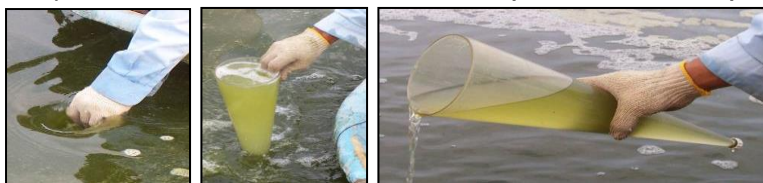
Fotos 44 e 45 – Esquema ilustrativo com cones Imhoff sendo utilizados para mensurar os sólidos sedimentáveis Fonte: SCOPEL, Bruno - 2013.
